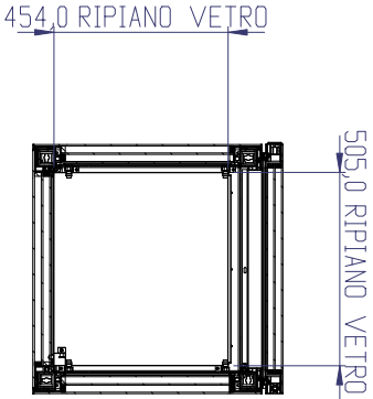
SEZIONE C-C
